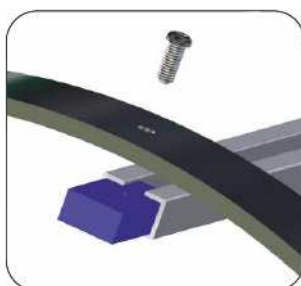
Fissaggio regolabile degli anelli gabbia mediante cavallotti in acciaio INOX e rondelle in nylon auto-lubrificante !
